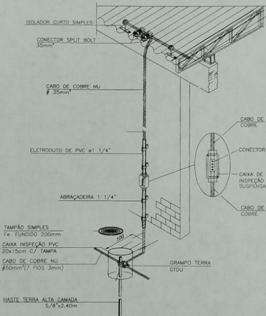
DETALHE DA INSTALAÇÃO DAS DESCIDAS
